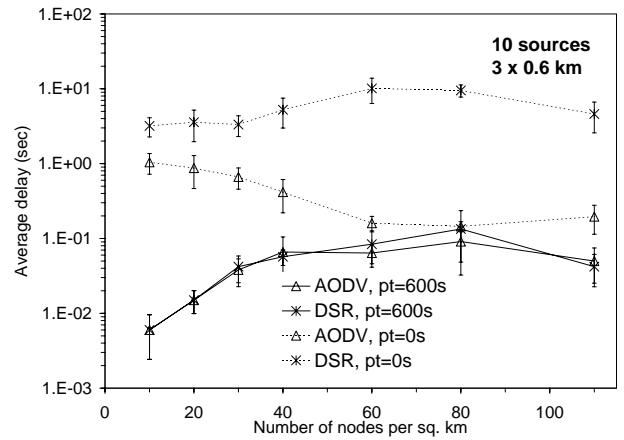
(d) Delay, 3 \times 0.6 \text{ km}^2
